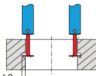
测量孔内凹槽直径 (凹槽深度 h_2 \leq 7\text{mm} )
