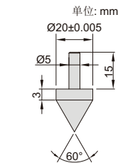
圆锥形测头(不锈钢)
